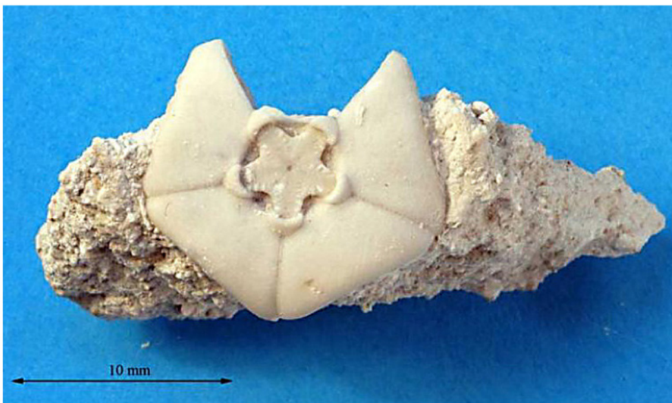
DK481. Soliljebæger af slægten Nielsenicrinus . Bryozokalk, Tidlig Danien, Sangstrup Klint. Finder: Niels Rask Petersen.
